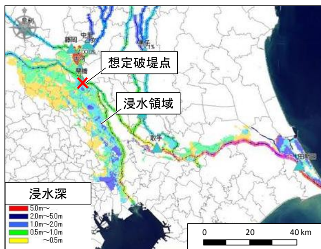
図 4: 栗橋付近を想定破堤点とする浸水域
