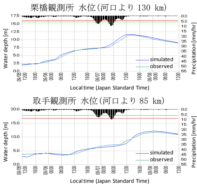
図 3: 2007 年台風 9 号再現シミュレーション
